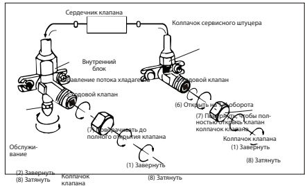
Присоединить к наружному блоку
